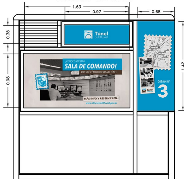
LATERAL DERECHO
