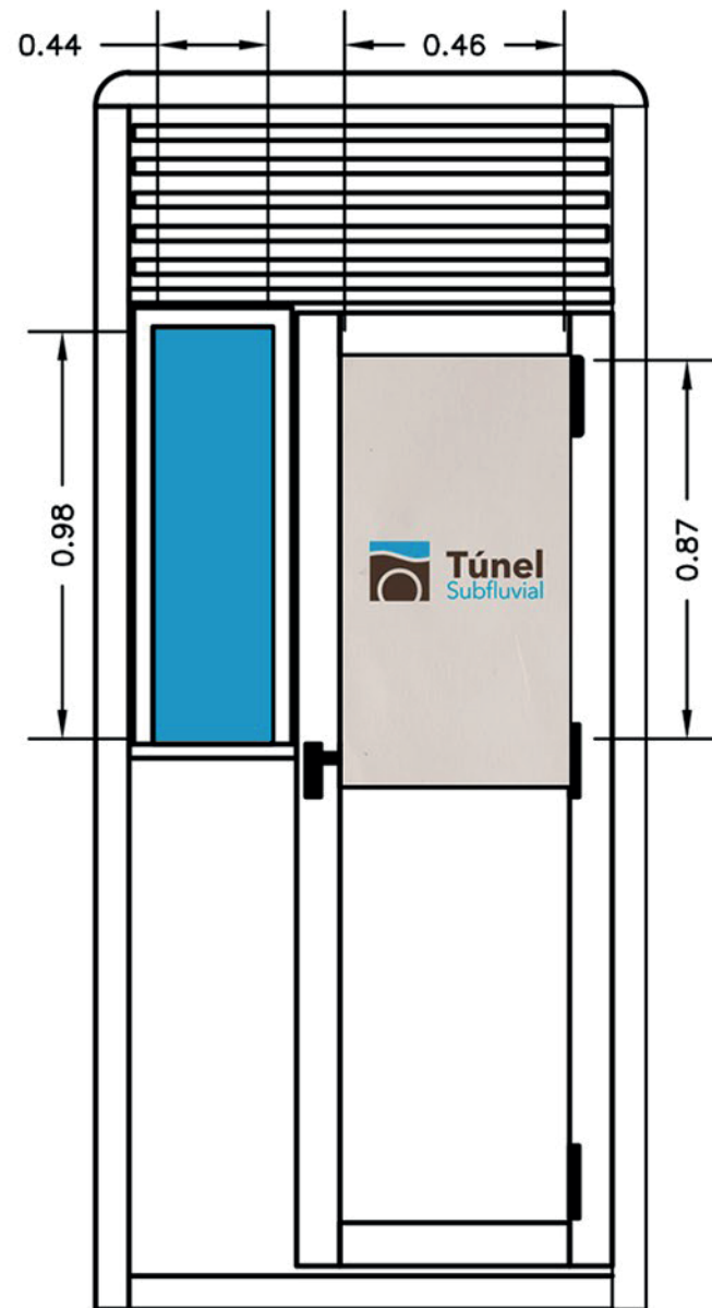
VISTA POSTERIOR
